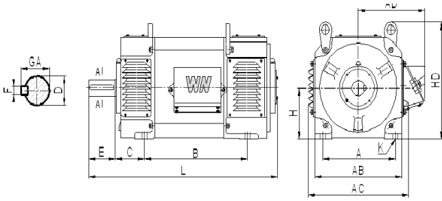
卧式、机座带底脚
