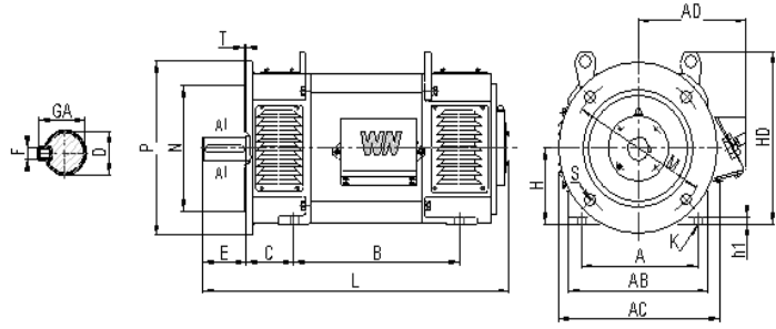
卧式、机座带底脚，端盖带凸缘
